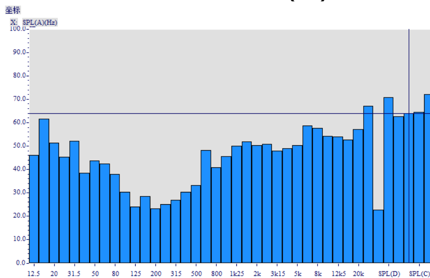
倍频段频谱图 Octave-Band(1m)
